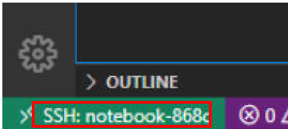
图 5-46 连接成功
