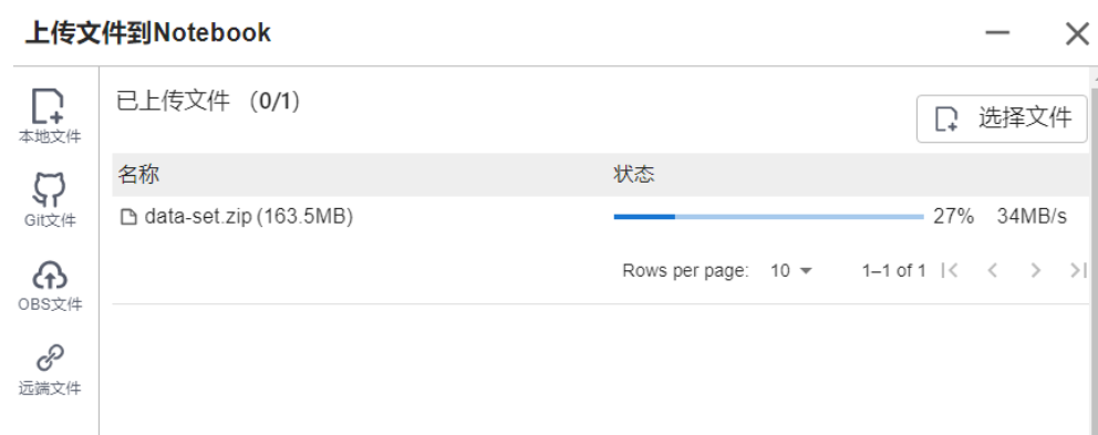
图 4-61 上传文件
