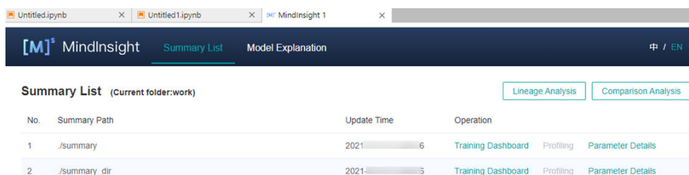
图 4-35 MindInsight 界面 ( 2 )
