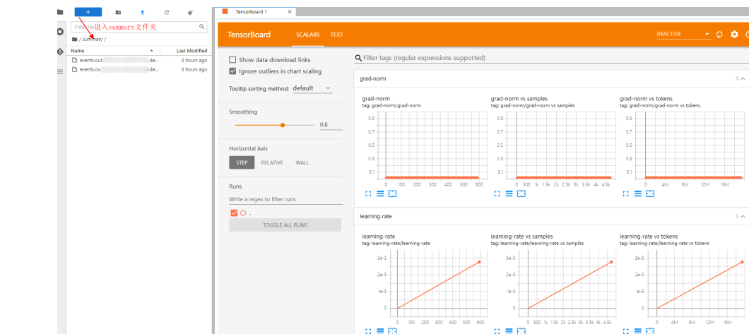
图 4-43 TensorBoard 界面（1）
